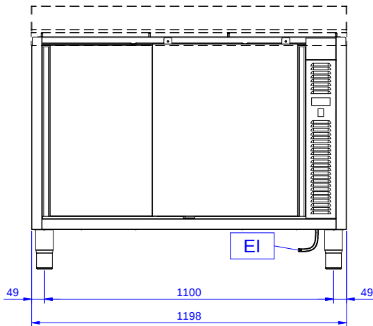
Alzado
